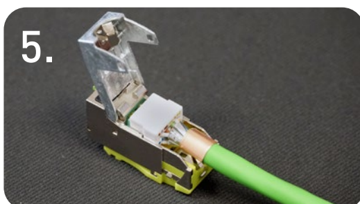
Wiremanager in das Modul einsetzen und Klappe schliessen.
