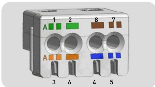
Wiremanager mit Farbcode nach TIA/EIA 568 Version A.
