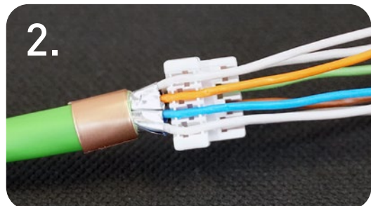
Adern in den Wiremanager entsprechend Farbcode einführen. Achtung: Wiremanager bündig an Folienschirme schieben.
