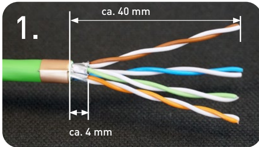
GREENforMEDIA Kabel vorbereiten
