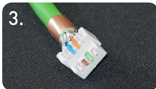
Überstehende Adern bündig abschneiden.
