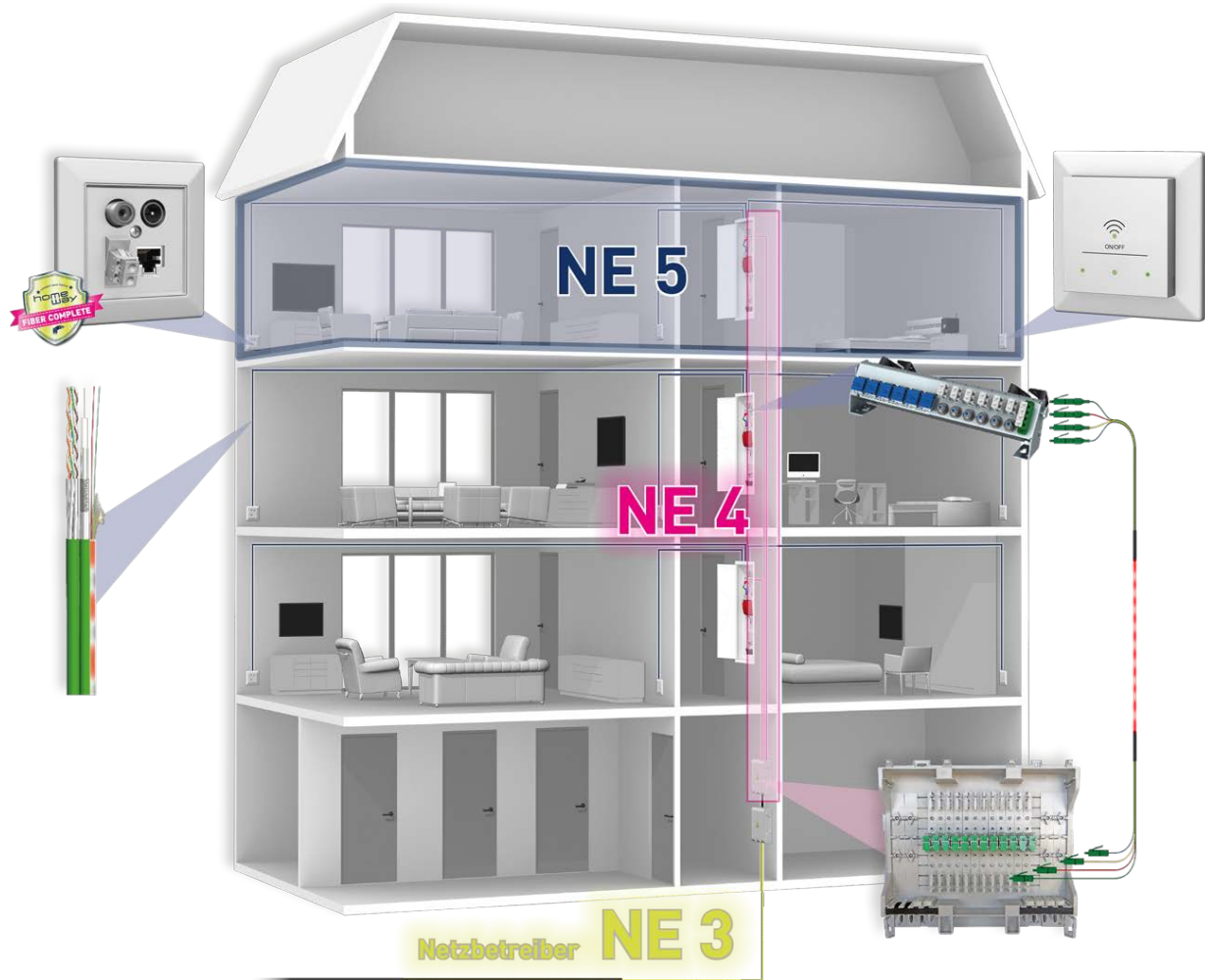
Multimedia-Inhouse-Netz mit fiberway (Netzebene 4) und in der Wohnung (Netzebene 5) mit System one.fiber
