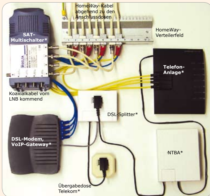
Abb.2: Beispiel für zentrale Verschaltung der aktiven Komponenten
